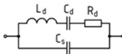
Рис.4. Еквівалентна схема ОАХ – генератору
