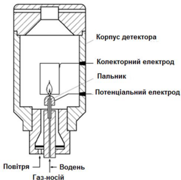
Рис. 3. Схема Полум'яно-іонізаційного детектору
